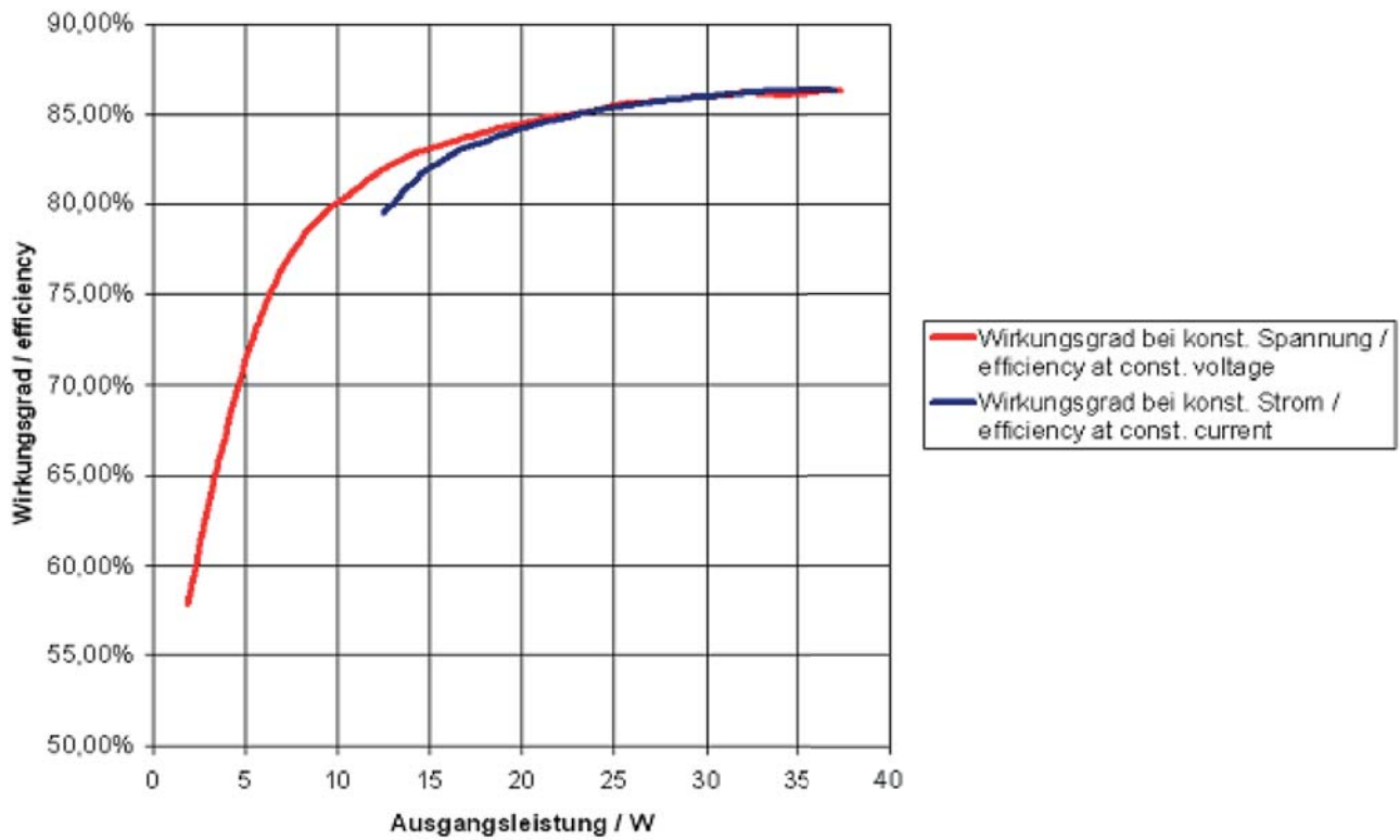
Wirkungsgrad über Ausgangsleistung / efficiency vs output power
