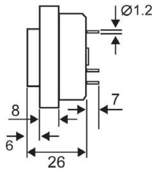
Seitenansicht / Side View
