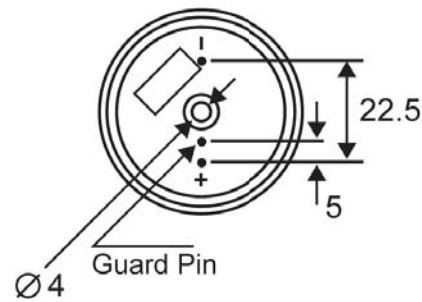
Untenansicht / Bottom View
