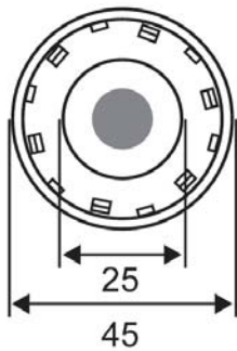
Frontansicht / Top View
