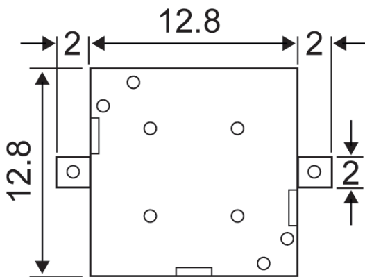
Frontansicht / Top View
