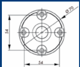
Montagefuß für ST 70 / 40
