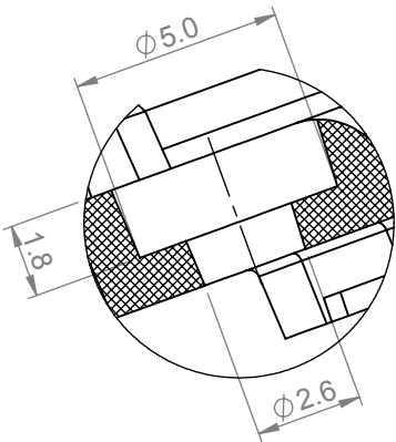
DETAIL Y SCALE 5 : 1
