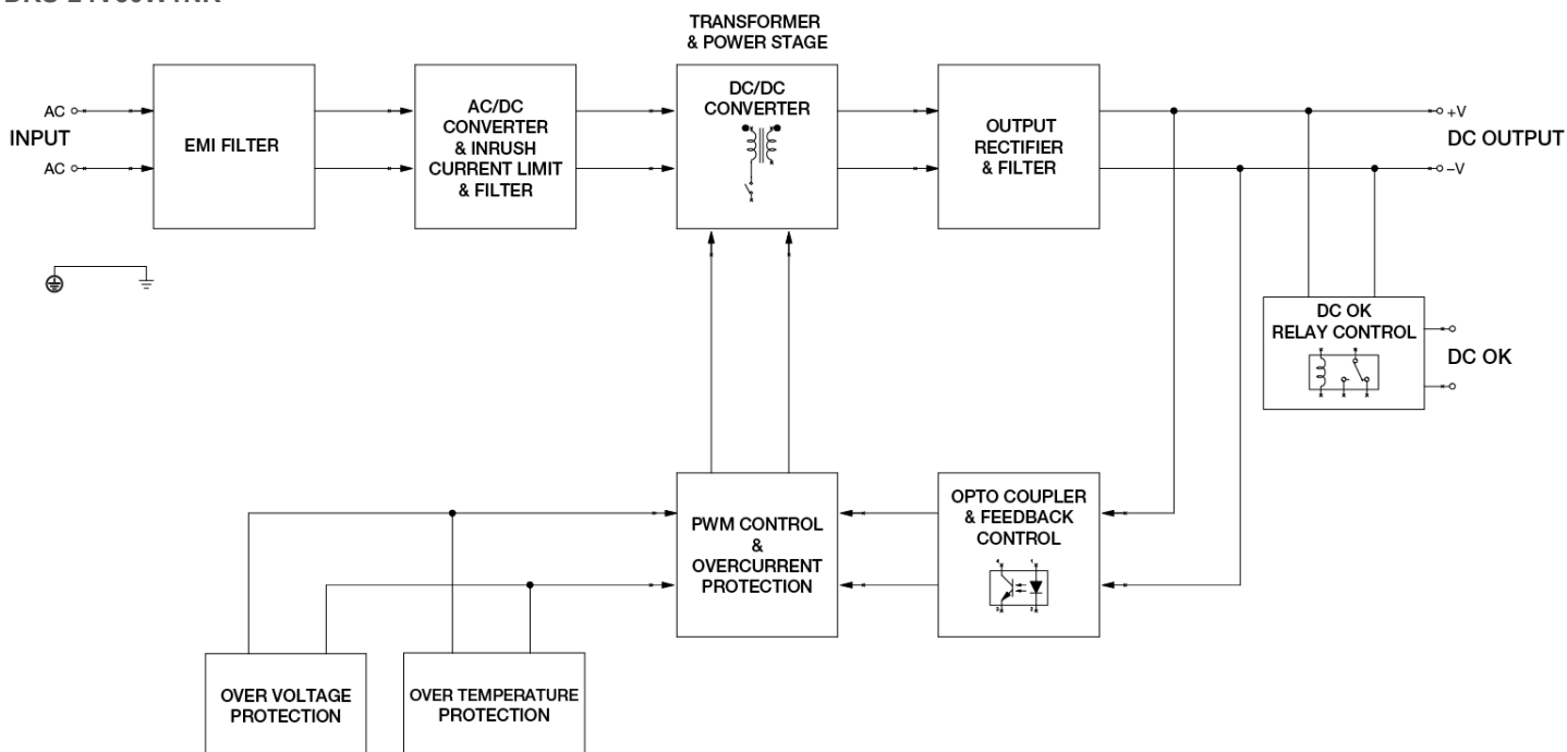
DRS-24V50W1NR
