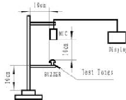
Test Equip
