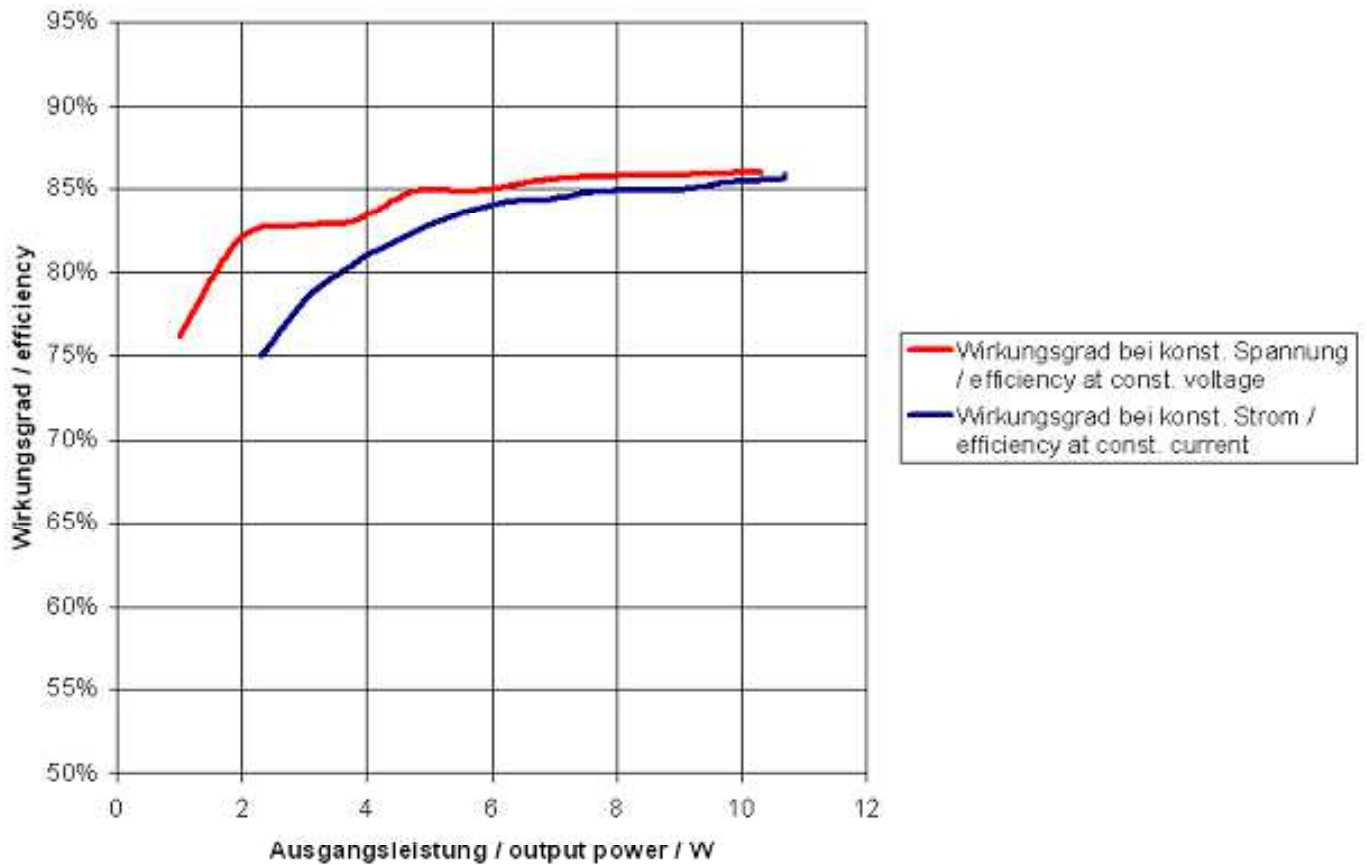
Wirkungsgrad über Ausgangsleistung / efficiency vs output power
