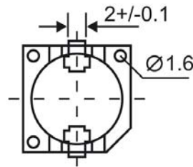
UNTENANSICHT / BOTTOM VIEW
