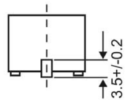
SEITERNANSICHT / SIDE VIEW 2
