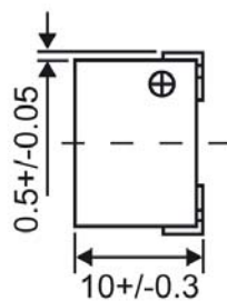
SEITERNANSICHT / SIDE VIEW 1
