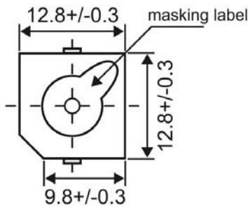
DRAUFSICHT / TOP VIEW
