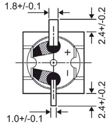
Untenansicht / Bottomview
