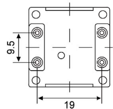
Untenansicht / Bottom View
