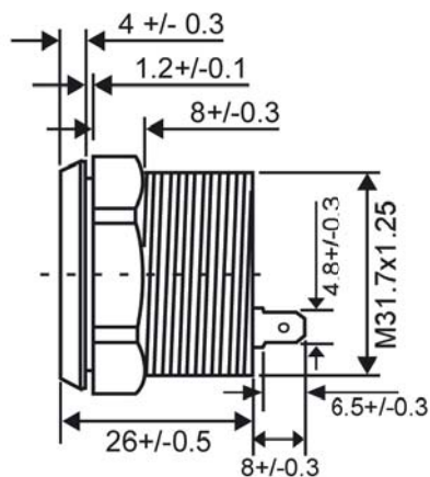
Seitenansicht / Side View
