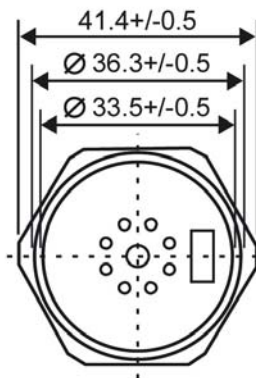
Frontansicht / Top View
