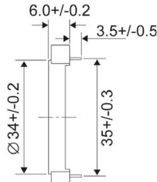
Seitenansicht/ Side View
